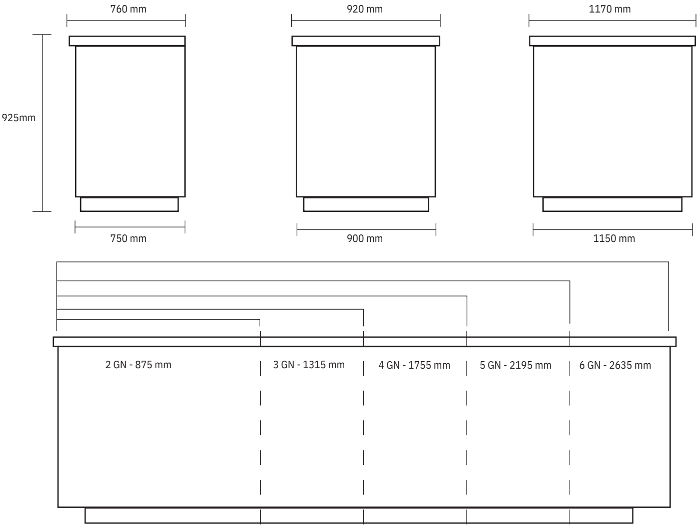
Modulo di testa - Head module
