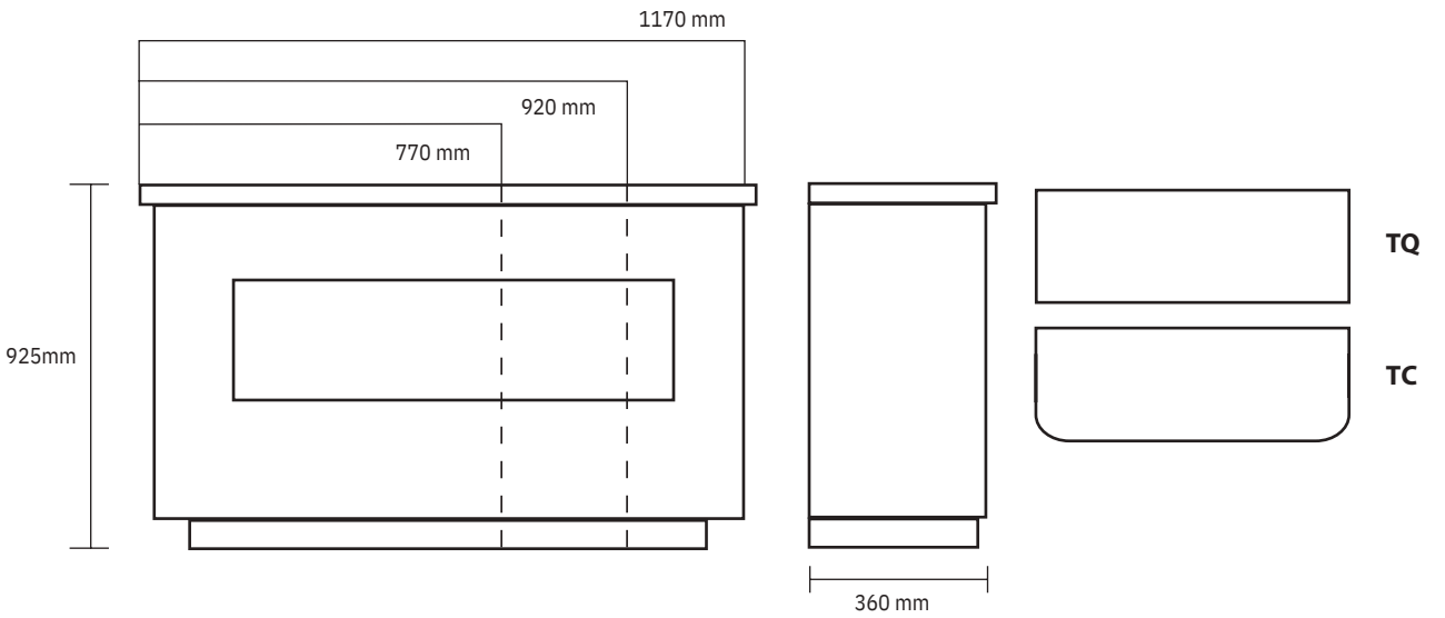
Modulo di testa - Head module
