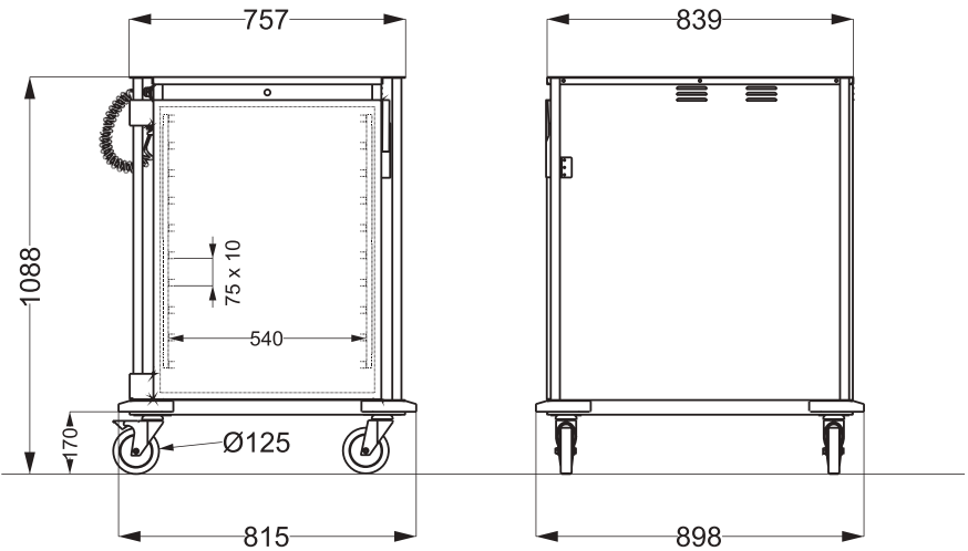
C 10 Profilo per vasche GN Profile for GN pans
