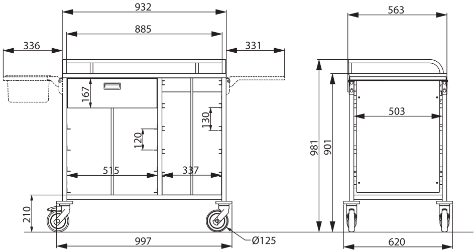
Nuovo cassetto con fondo pieno New drawer with full bottom
